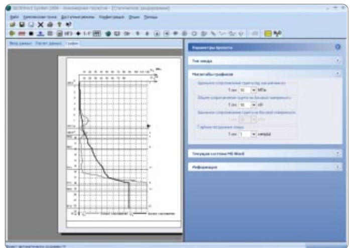
Графики статического зондирования в GeoniCS Инженерная геология (GeoDirect)
