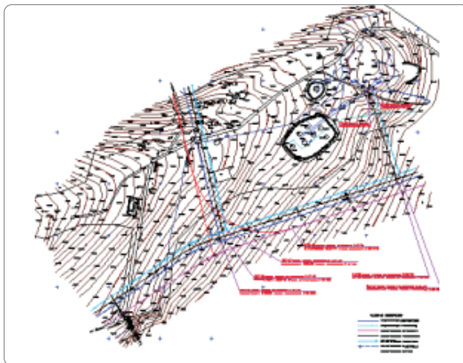
План площадки
