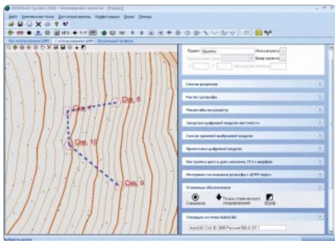
Нанесение скважин и линий разрезов с использованием ЦММ в GeoniCS Инженерная геология (GeoDirect)
