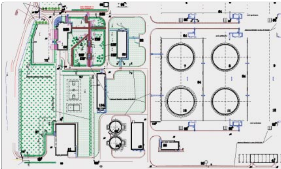
Город Приморск: план благоустройства
