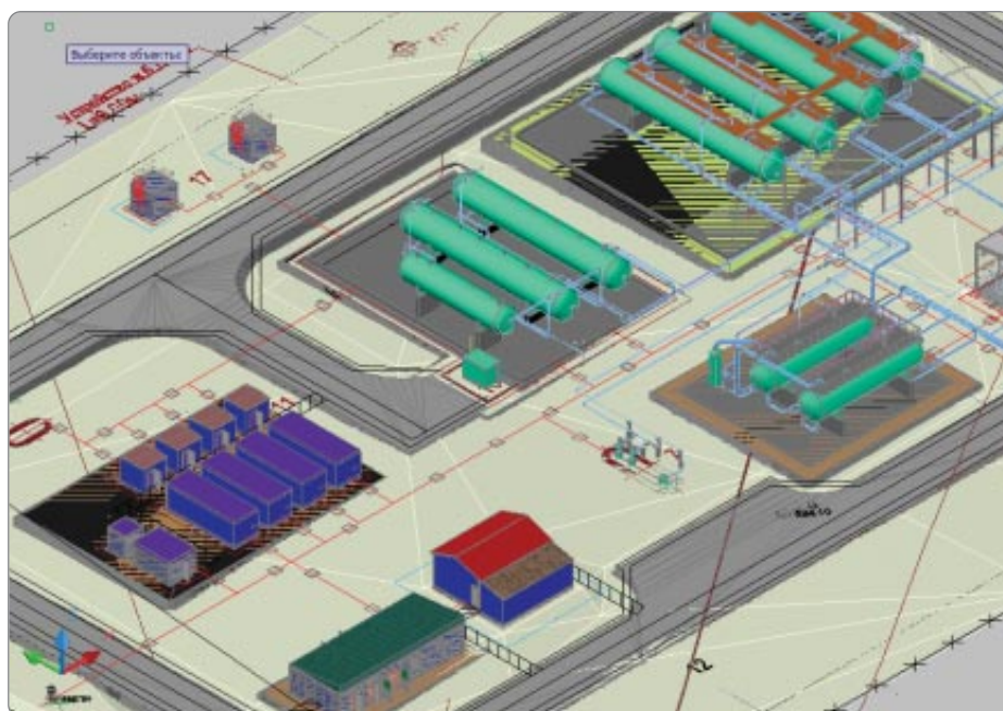
Трехмерная поверхность площадки, полученная в GeoniCS, и расположенное на ней оборудование, созданное в другой программе технолого-монтажным отделом
