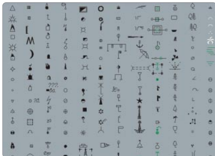
Точечные условные знаки
