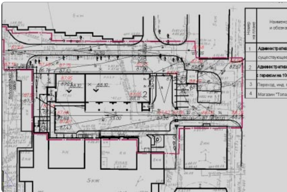
План организации рельефа
