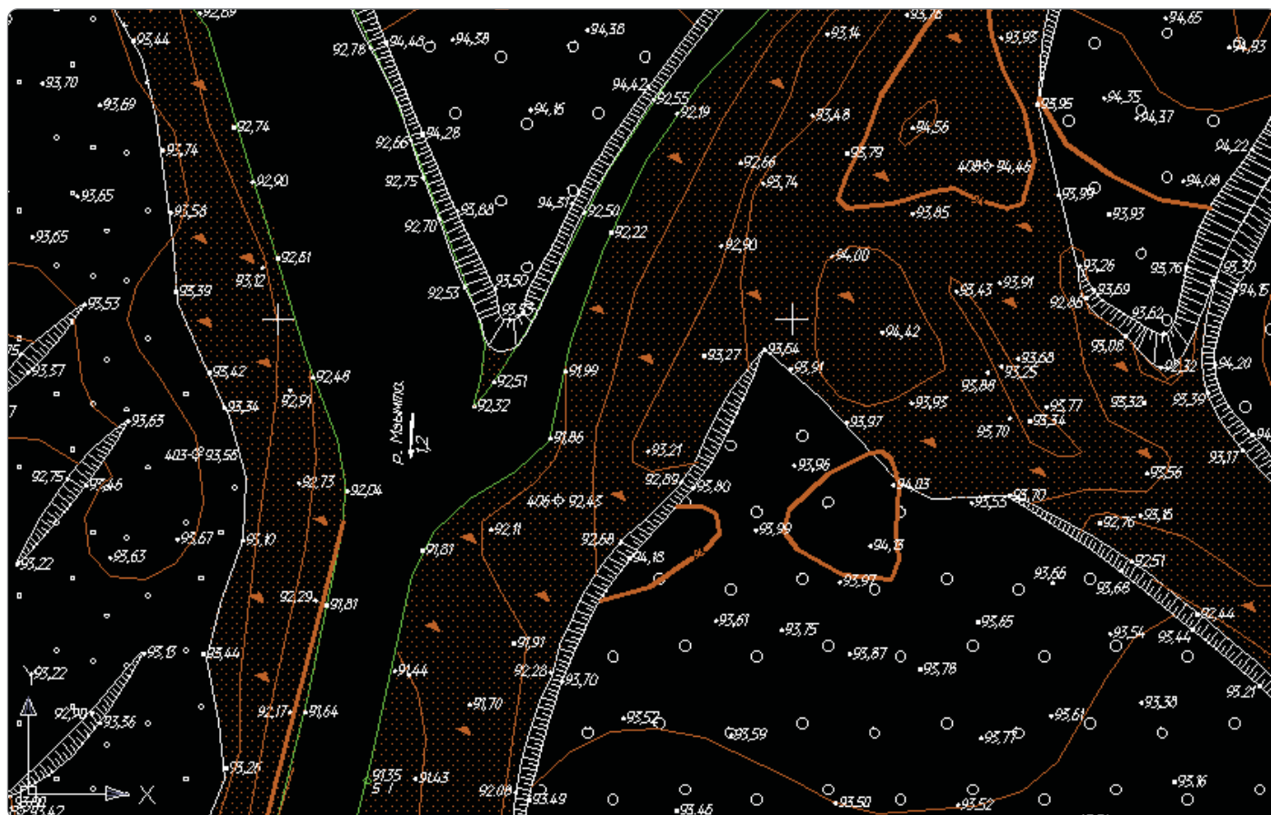
Участок топосъемки реки Мзымта
