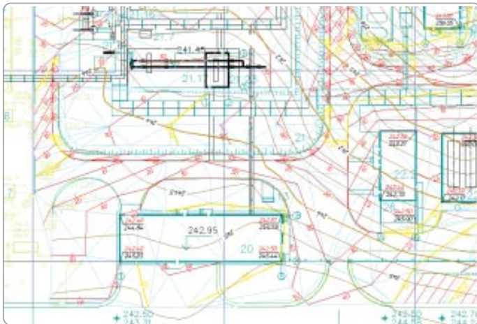
Вертикальная планировка
